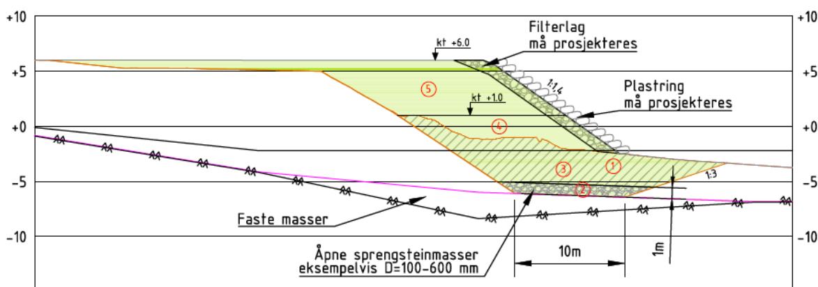
Figur 5-1: Prinsipsnitt mudring og utfylling ved profil M-M.
