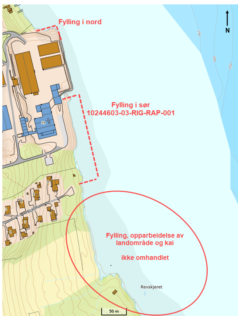
Figur 1-1: Skisse over de ulike områdene som skal utvikles i prosjektet. Dette dokumentet omhandler kun geoteknisk prosjektering og fyllingsprosedyrer for utførelse av fyllingen i nord.
